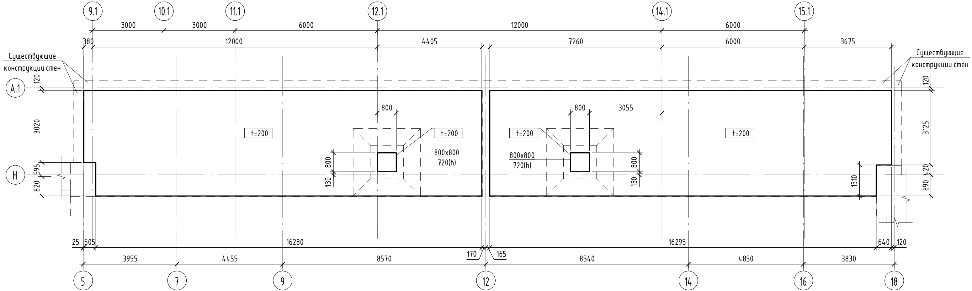
Схема расположения плиты по грунту ФПм-3 в осях 5-18/Н-А.1
