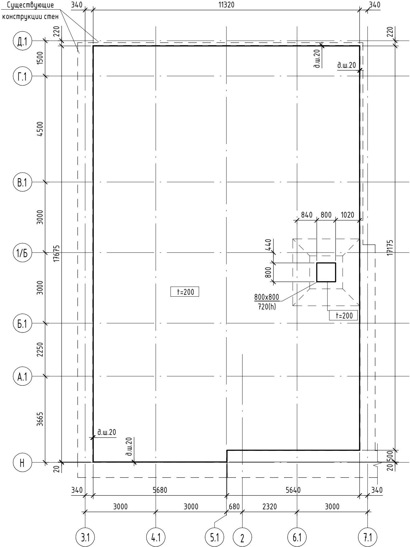
Схема расположения плиты по грунту ФПм-2 в осях 3.1-7.1/Н-Д.1
