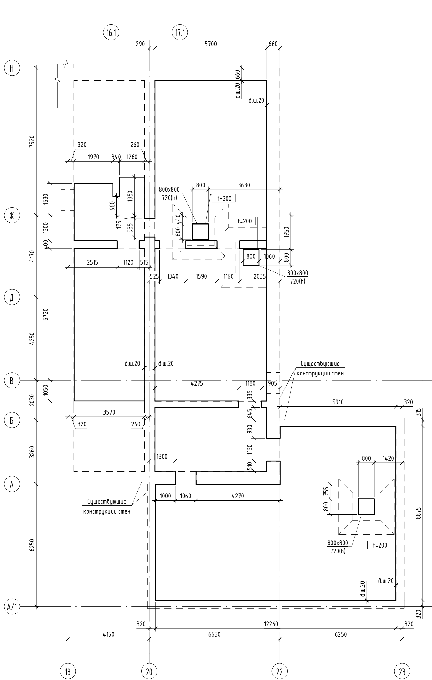
Схема расположения плиты по грунту ФПм-4 в осях 18-23/А1-Н
