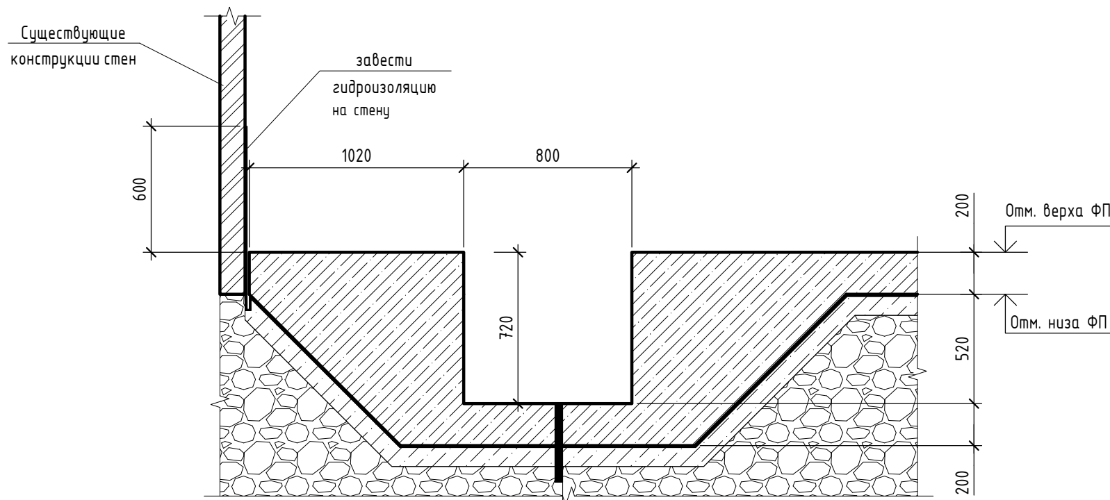
Узел устройства гидроизоляции в зоне приямка
