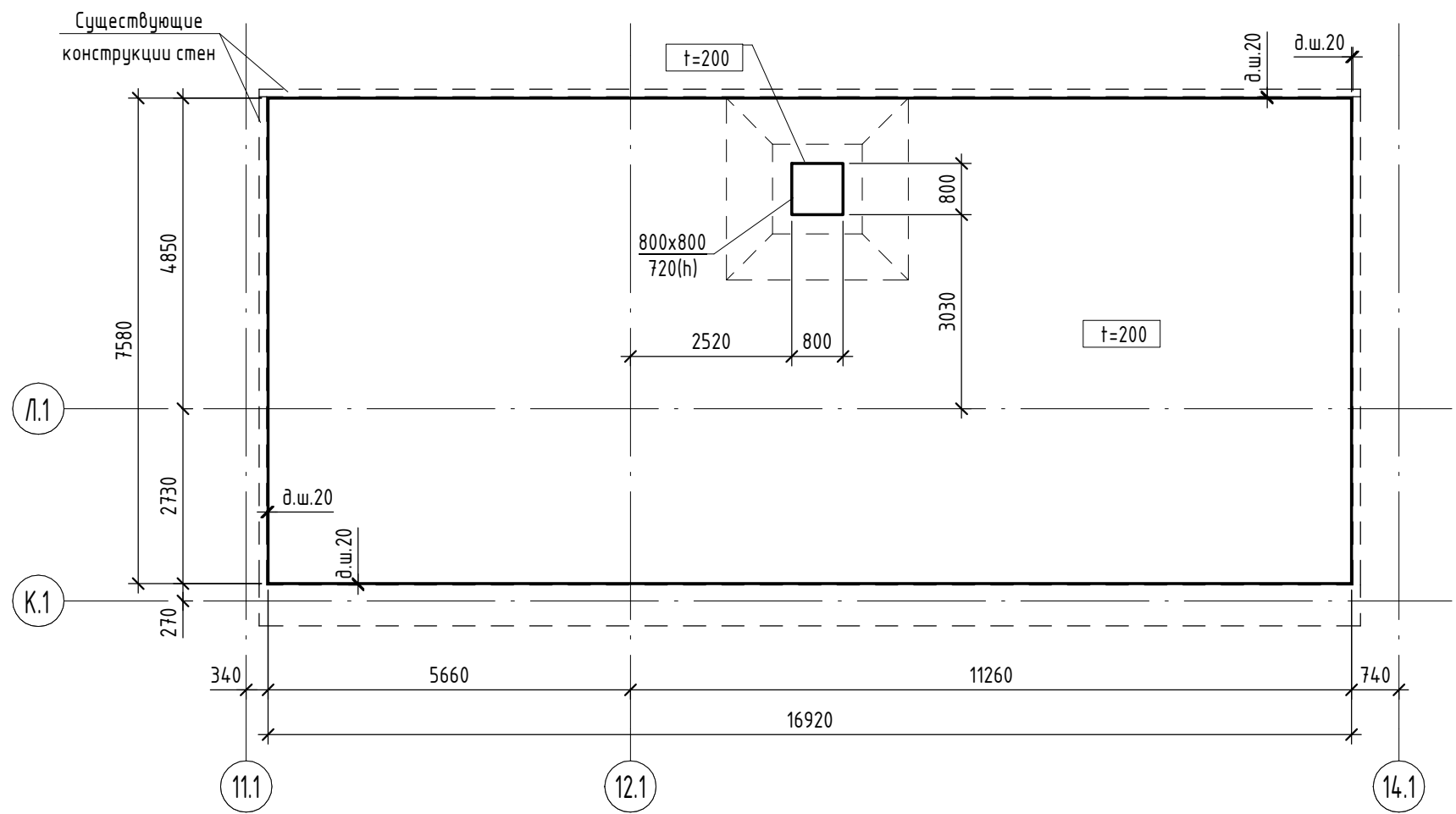
Схема расположения плиты по грунту ФПм-1 в осях 11.1-14.1/К.1-Л.1
